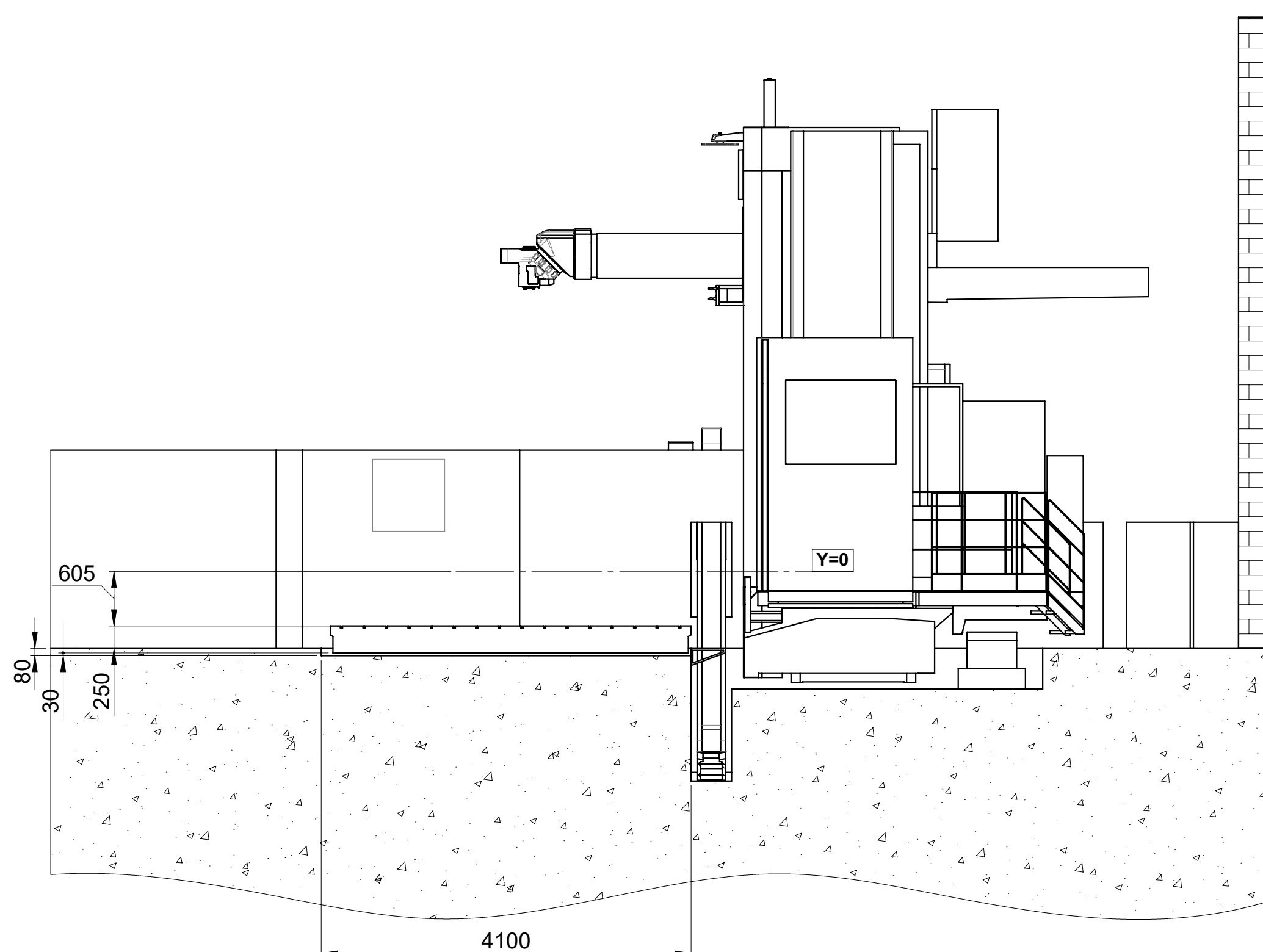
ELEMENTO FRONTALE N°3 PIANO FISSO / FLOOR PLATE 2000X4000
